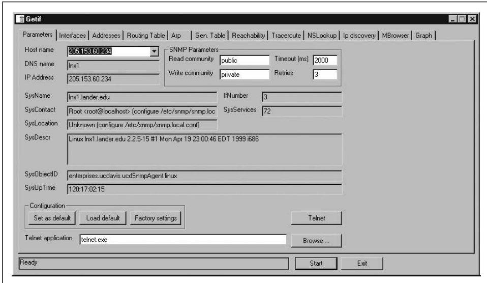
Figure 7-14. getif Parameters tab
